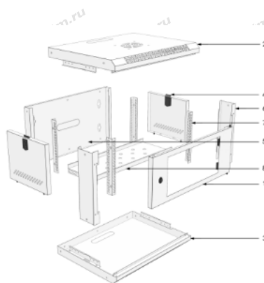
Рис.1. Порядок сборки шкафа
