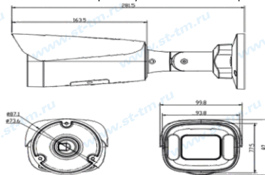
Рис.4 Габаритные размеры видеокамеры
