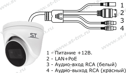
Рис.1 Схема подключения видеокмеры
