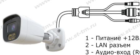
Рис. 1 Схема подключения видеокамеры
