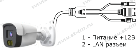
Рис. 1 Схема подключения видеокамеры
