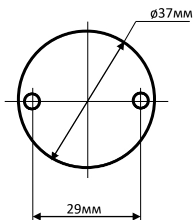
Монтажный чертёж
