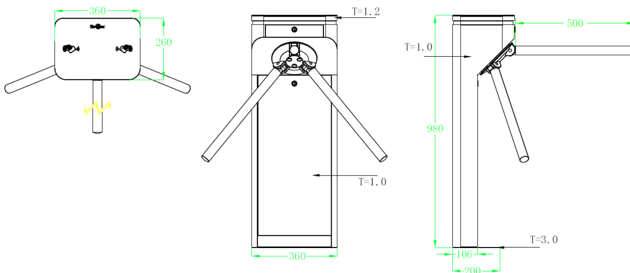
Рисунок 1. Габаритные размеры турникета
