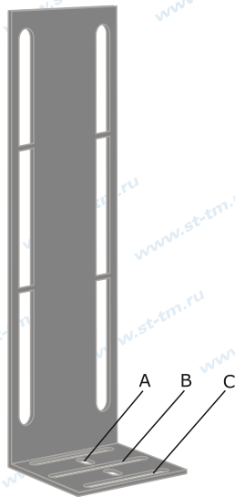
А - 8x4 мм; В - 40x4 мм; С - 34x4 мм
