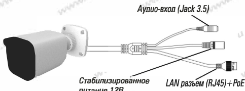
Рис.1 Схема подключения
