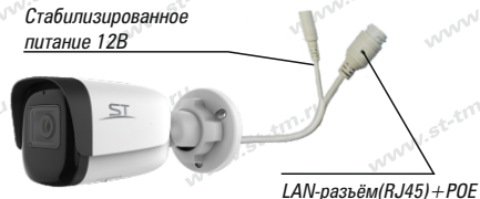
Рис.1 Схема подключения видеокamеры
