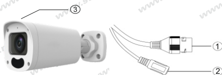
Рис.1 Схема подключения видеокamеры
