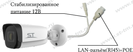
Рис.1 Схема подключения видеокamеры
