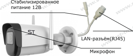
Рис.1 Схема подключения видеокamеры
