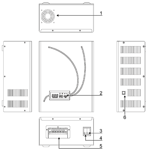
Рисунок 1. Внешний вид стабилизаторов напряжения SMARTWATT AVR SERVO 5000-10000SW. Описание элементов приводится в таблице 1.
