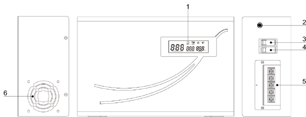
Рисунок 4. Внешний вид стабилизаторов напряжения SMARTWATT AVR SLIM 8000-12000VA. Описание элементов приводится в таблице 4.
