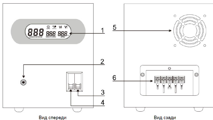
Рисунок 1. Внешний вид стабилизаторов напряжения SMARTWATT AVR STRONG 15000-20000VA. Описание элементов приводится в таблице 1.
