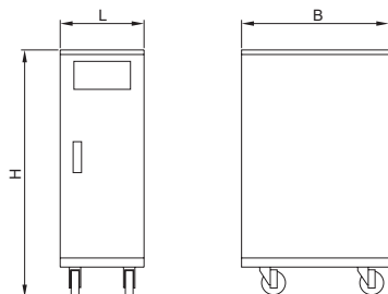
Рисунок 1 – Габаритные размеры стабилизатора / Figure 1 – Overall dimensions of the stabilizer
