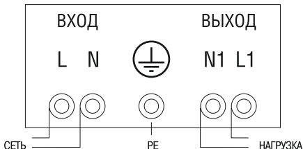
Рис 3. Схема подключения стабилизаторов от 3 до 12 кВА
