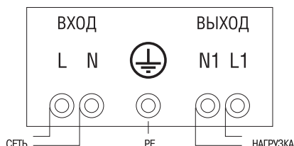
Рисунок 3 – Схема подключения стабилизаторов от 3 до 12 кВА.
