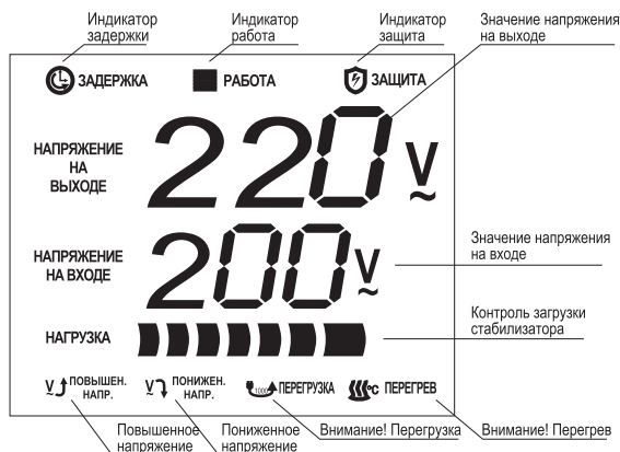
Рисунок 2 – Индикация режимов работы стабилизаторов
