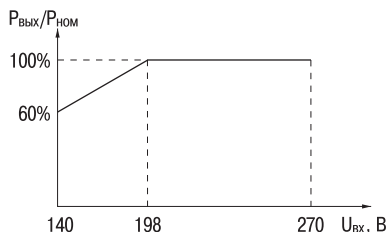
Рисунок 1 – Зависимость выходной мощности от входного напряжения, где U_{вх} – входное напряжение, P_{вых} – выходная мощность, P_{ном} – номинальная (паспортная) выходная мощность
