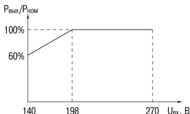
Рисунок 1 – Зависимость выходной мощности от входного напряжения, где
