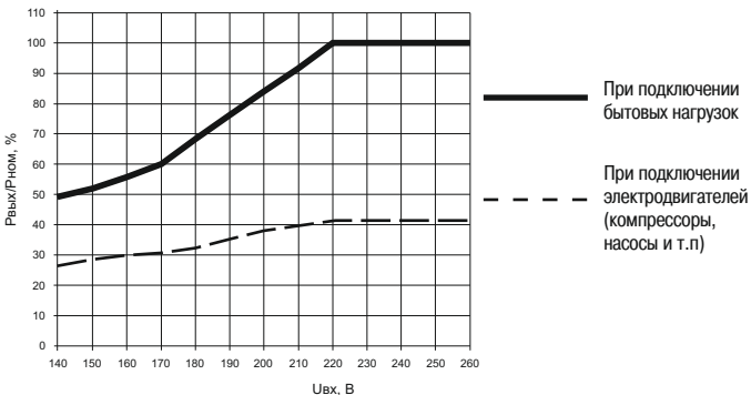
Рисунок 2 – Зависимость выходной мощности стабилизатора от входного напряжения
