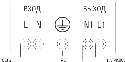
Рис 4. Схема подключения стабилизаторов
