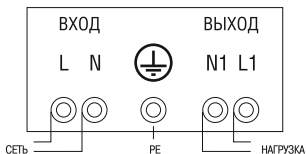
Рисунок 5 – Схема подключения стабилизаторов
