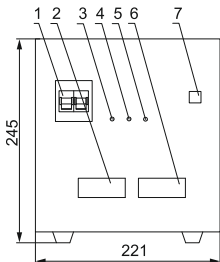
Рисунок 2 – Передняя панель стабилизатора
