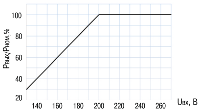
Рисунок 1 – Зависимость выходной мощности от входного напряжения
