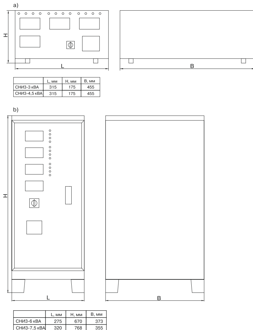
Рисунок 1 – Габаритные размеры: а) СНИИЗ-3 кВА; СНИИЗ-4,5 кВА; б) СНИИЗ-6 кВА; СНИИЗ-7,5 кВА
