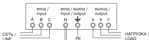
Рисунок 7 – Схема подключения СНИЗ от 6 до 7,5 кВА
