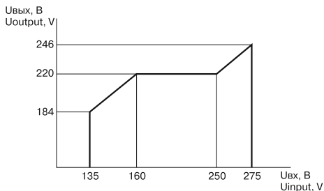
Рисунок 5 – Зависимость величины однофазного выходного напряжения стабилизатора при изменении входного напряжения без нагрузки
