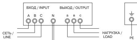
Рисунок 6 – Схема подключения СНИЗ-3 кВА
