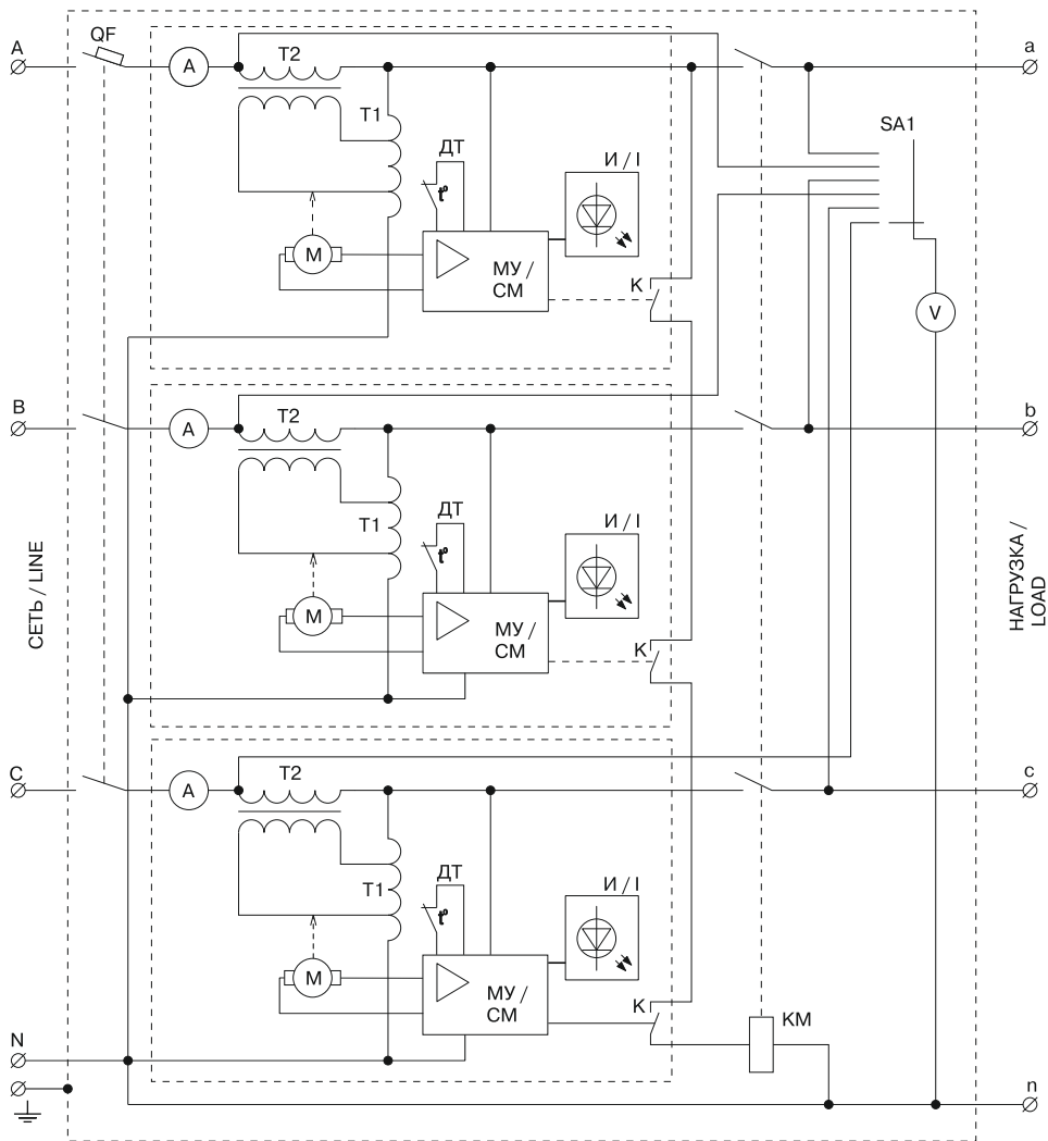
Рисунок 4 б – Структурные схемы стабилизаторов: СНИЗ-15 кВА; СНИЗ-20 кВА; СНИЗ-30 кВА; СНИЗ-45 кВА; СНИЗ-60 кВА с дополнительным вольтодобавочным трансформатором
