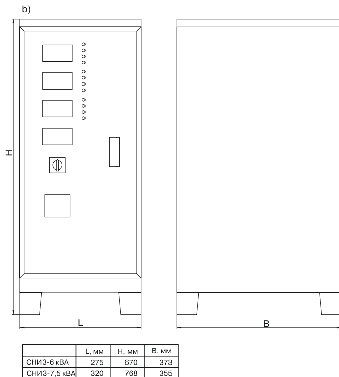
Рисунок 1 – Габаритные размеры: а) СНИИЗ-3 кВА; СНИИЗ-4,5 кВА; б) СНИИЗ-6 кВА; СНИИЗ-7,5 кВА
