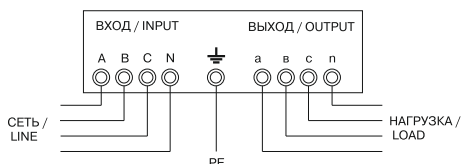
Рисунок 8 – Схема подключения СНИЗ от 15 до 60 кВА
