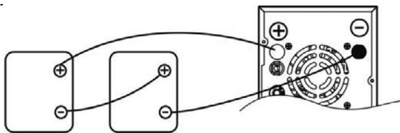
Рисунок 1. Пример подключения модели 1000 Online
