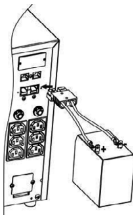
Рисунок 2. Подключение внешнего АКБ к ИБП
