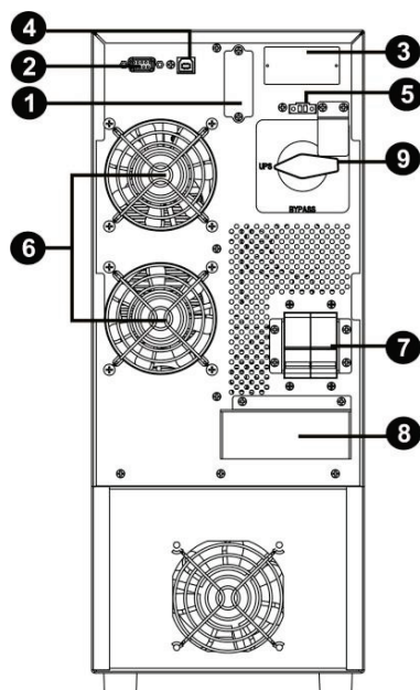
Рисунок 1: Задняя панель
