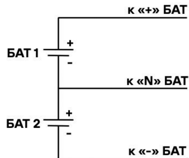
Схема подключения проводов аккумулятора
