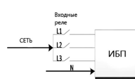
Схема входного реле для модели с одним входом
