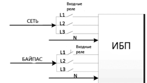
Схема входного реле для модели с двумя входами
