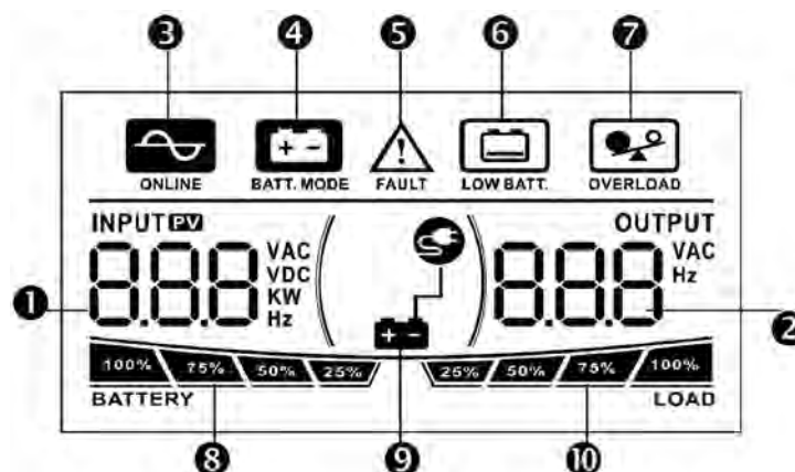
LCD экран
