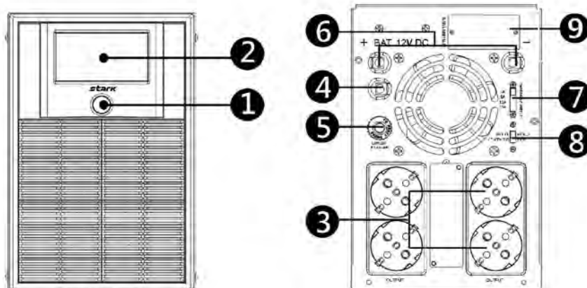
Вид спереди
