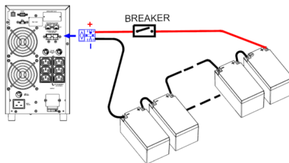
Рисунок 1. Пример подключения модели 2000 Online
