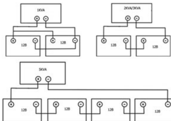
Рис. 3 Последовательное подключение внешних АКБ
