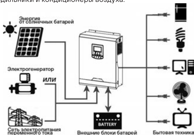
Рис. 1 Система электропитания
