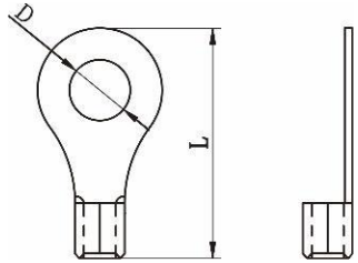
Кольцевой наконечник
