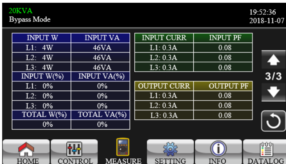
Экран измерения Страница 3
