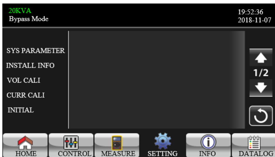
Меню настройки "Специалист по обслуживанию". Страница 1
