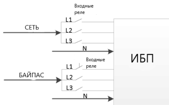
Схема входного реле для модели с двумя входами
