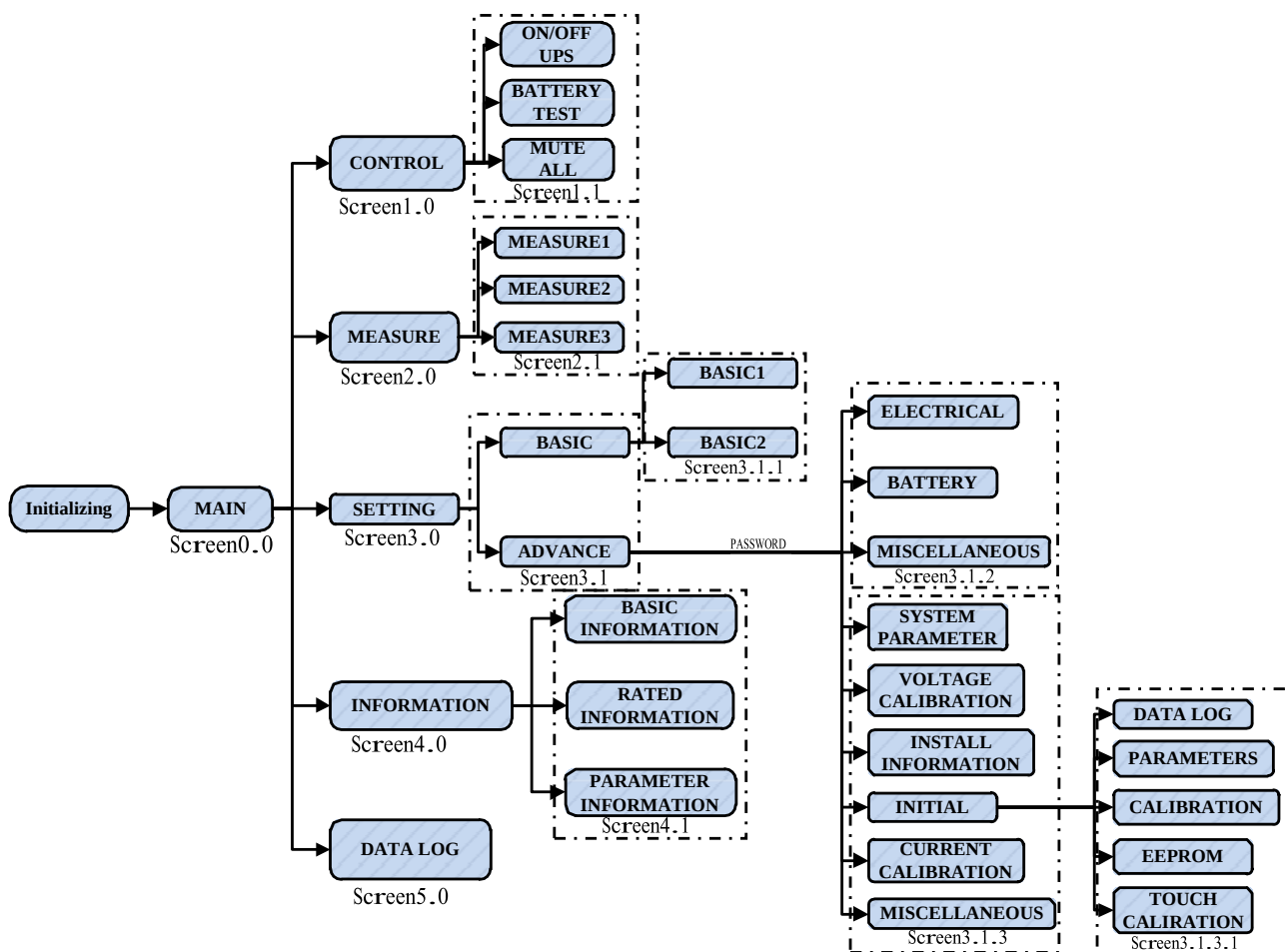
Рисунок - Разделы меню
