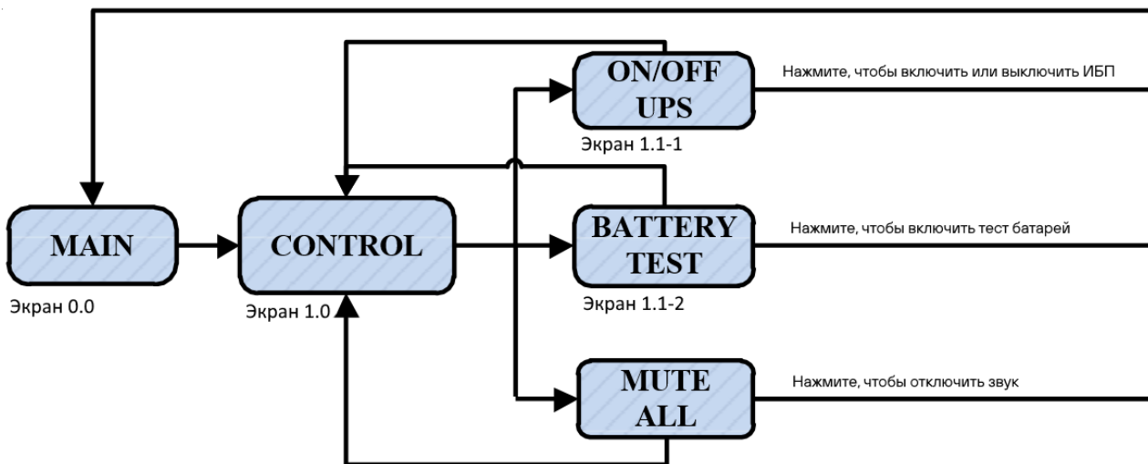
Рисунок - Экран 1.0. Древо раздела управления
