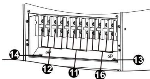
Клеммы Выход/Вход/Байпас 15000 ONLINE DUAL
