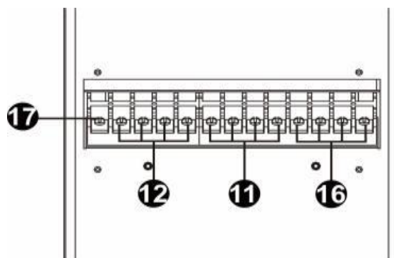
Клеммы Выход/Вход/Байпас 40000 ONLINE DUAL
