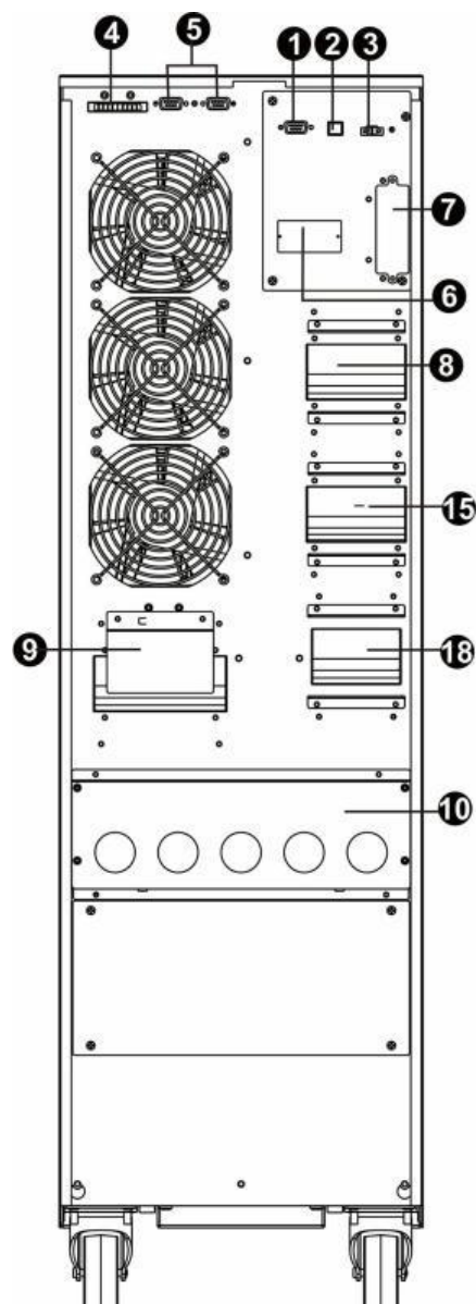
Задняя панель ИБП 40000 ONLINE DUAL
