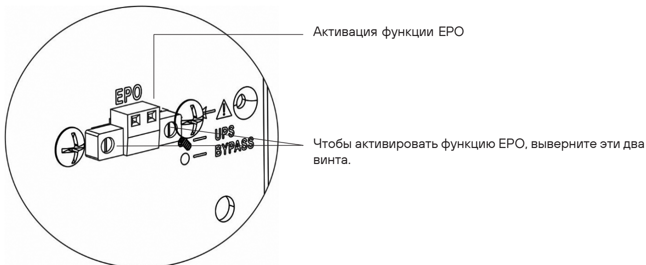
Рисунок 6 – Клемма аварийного отключения EPO
