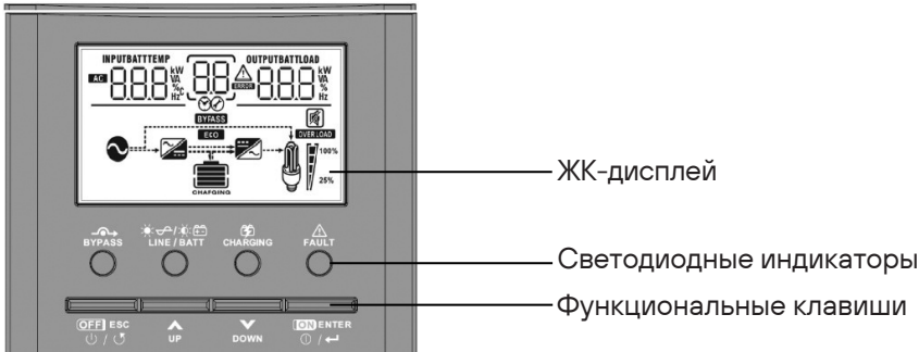
Рисунок 7 Панель управления
