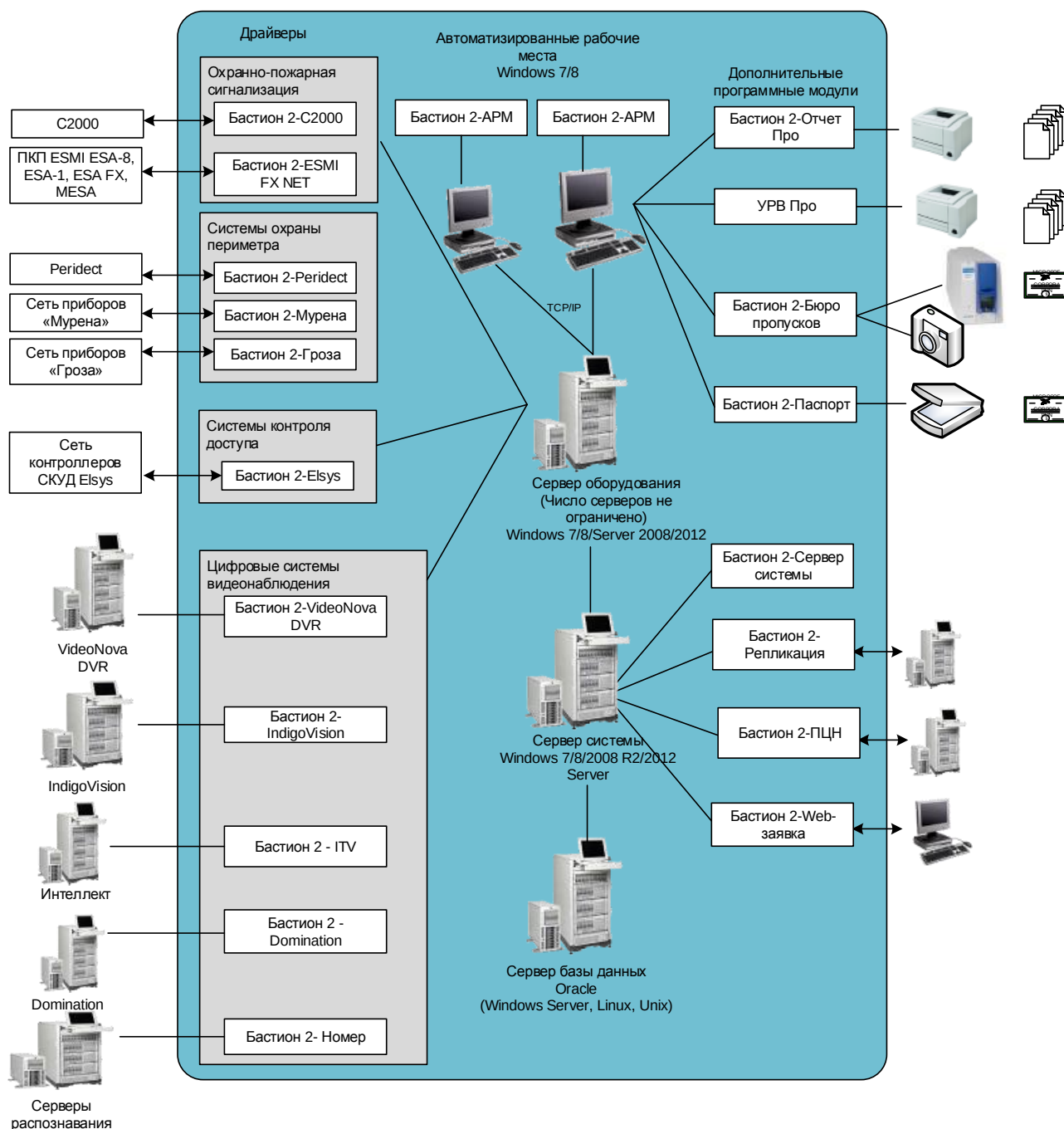
Рис. 2. Структура модулей АПК «Бастион-2»
