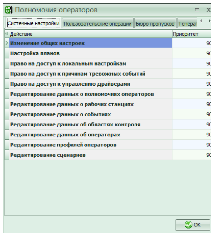
Рис. 9. Окно настройки полномочий пользователей
