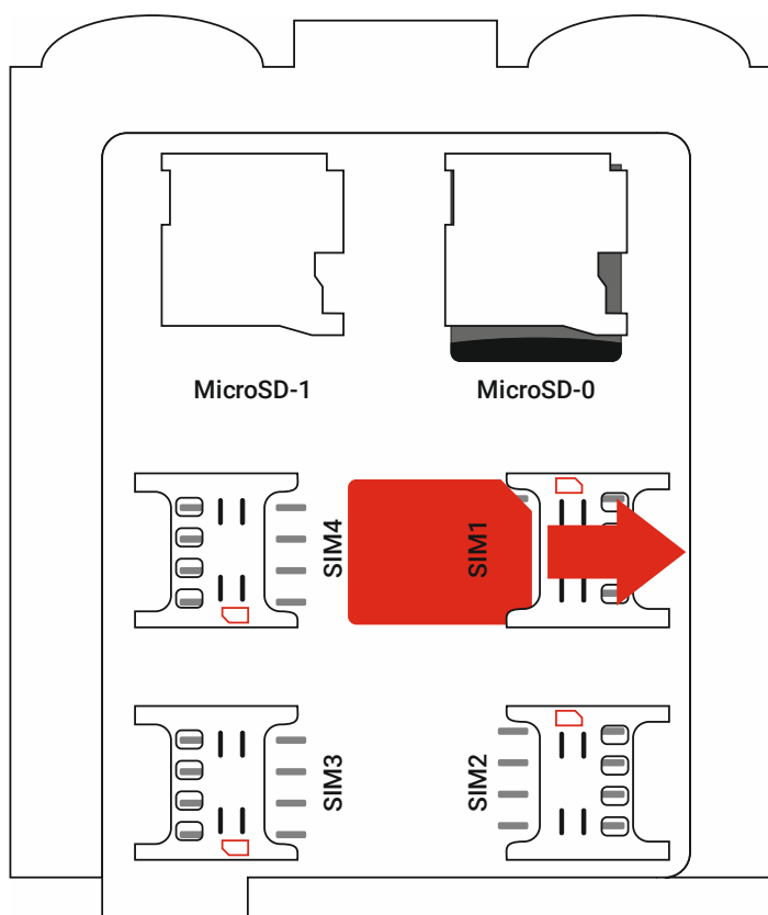
Рисунок 3. Установка SIM-карт
