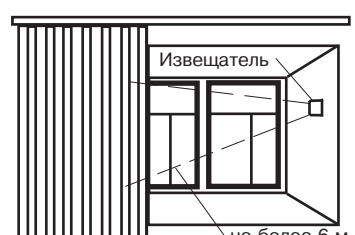
Рисунок 8 – Установка извещателя между стеклом и занавесями (жалюзи)
