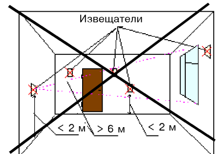
Рис. 7 - Не рекомендуемые места установки извещателя
