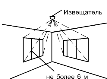
Рис. 5 - Установка извещателя на потолке (для блокировки оконных проемов в соседних стенах)
