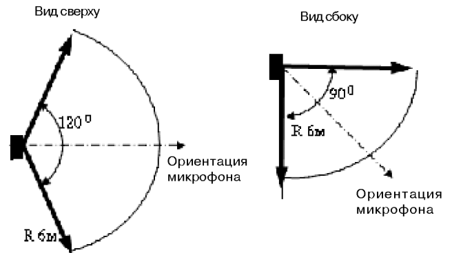
Рис. 1- Диаграмма зоны обнаружения АК-канала
