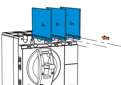
Рисунок 6 – Установка межполюсных перегородок на выключатель 4р
