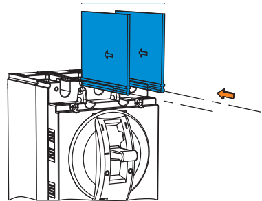
Рисунок 5 – Установка межполюсных перегородок на выключатель 3р
