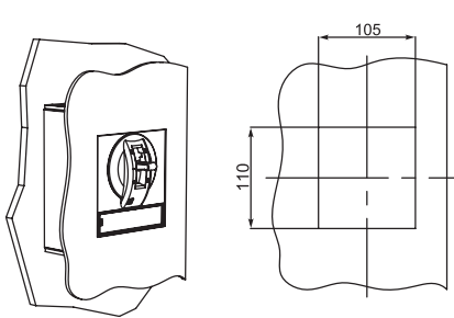
Рисунок 8 – Разметка для выреза панели OptiMat T250 3р
