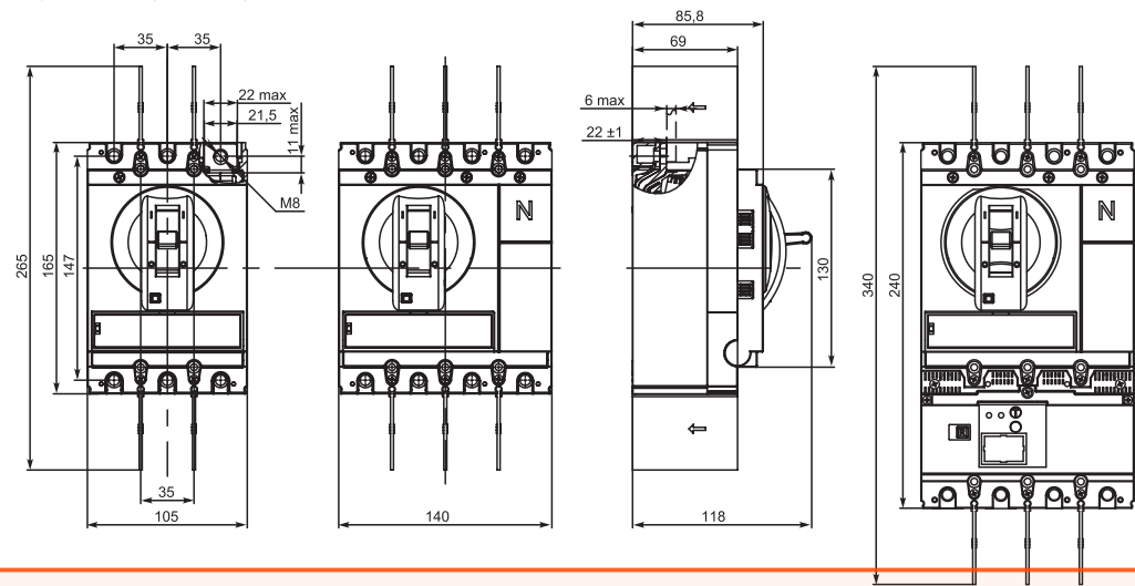
Рисунок 7 – Габаритный чертеж
