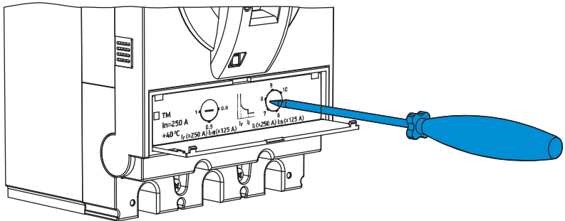
Рисунок 12 – Регулировка уставок терромагнитного расцепителя защиты
