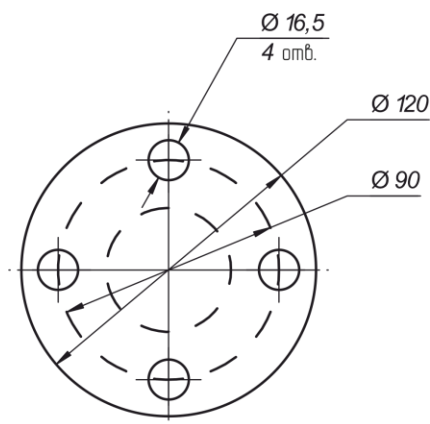
Рисунок 6. Разметка установочных отверстий
