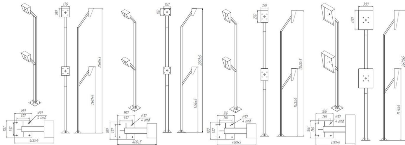
Двухуровневая Стойка для считывателя АЯКС 170x180, базовая, усиленная Двухуровневая Стойка для считывателя АЯКС 150x150, базовая, усиленная Двухуровневая Стойка для считывателя АЯКС 150x250, базовая, усиленная Двухуровневая Стойка для считывателя АЯКС 300x400, базовая, усиленная
