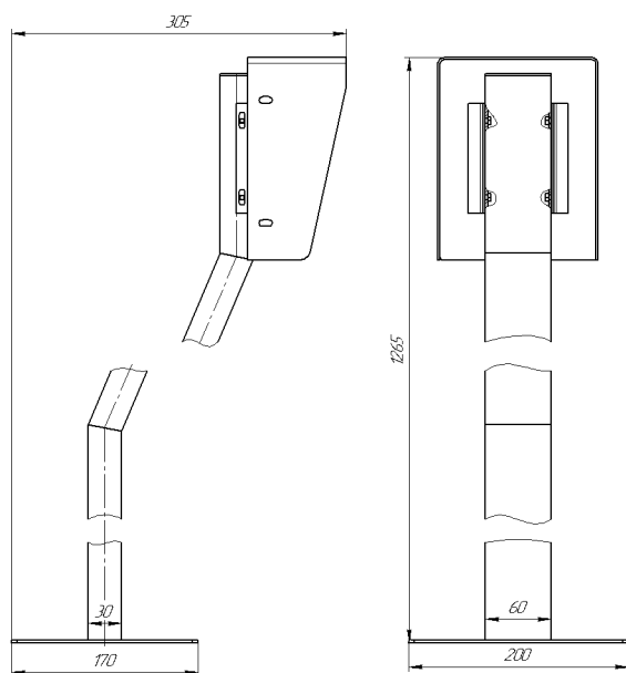
Рис.1 Стойка
