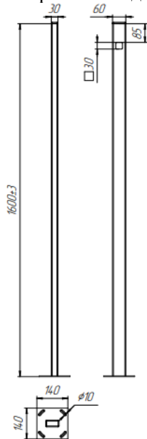
Рис.2 Стойка «Лайт»
