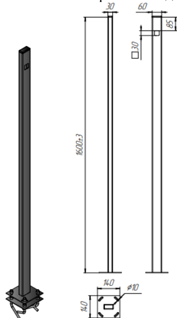
Рис.2 Стойка «Лайт»
