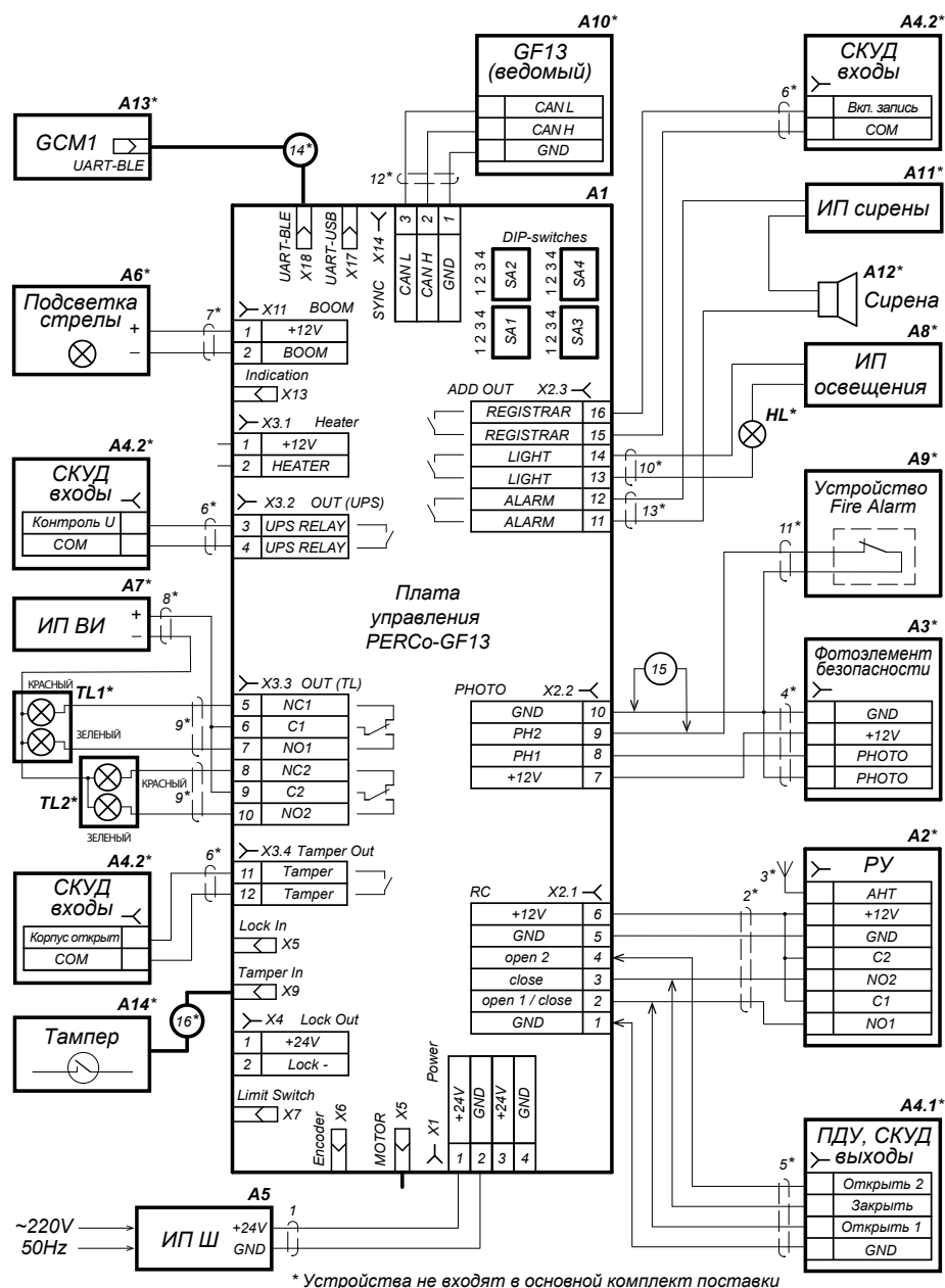
Схема электрических соединений слагбаума GF13
