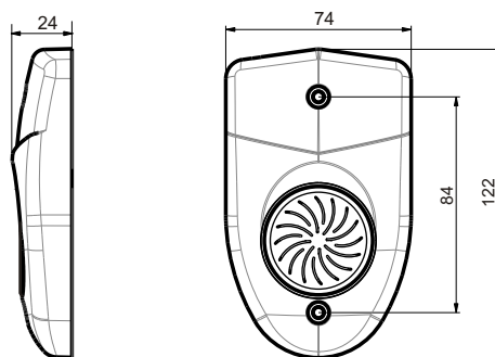
Рис.1. Габаритные и установочные размеры оповещателя
