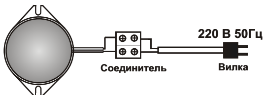
Рис.2 Схема подключения устройства “СБ-3”.
