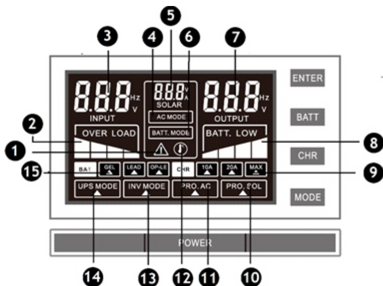
Рис.4 Индикаторы ЖК-дисплея
