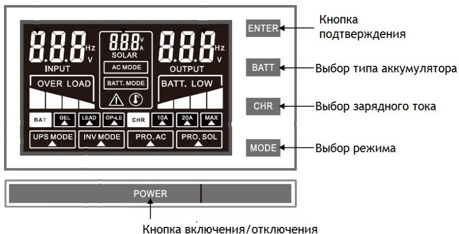
Рис.3 Панель управления
