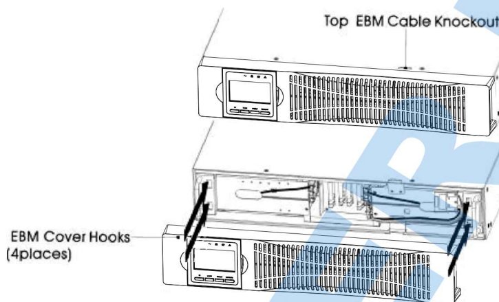
Рис. 3-11. Установка лицевой панели.
