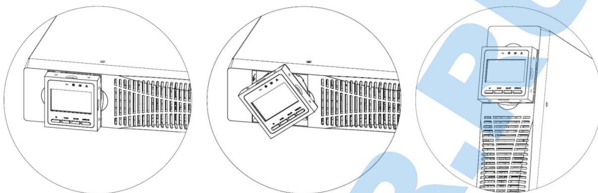
Рис. 3-6. Поворот ЖК-дисплея.
