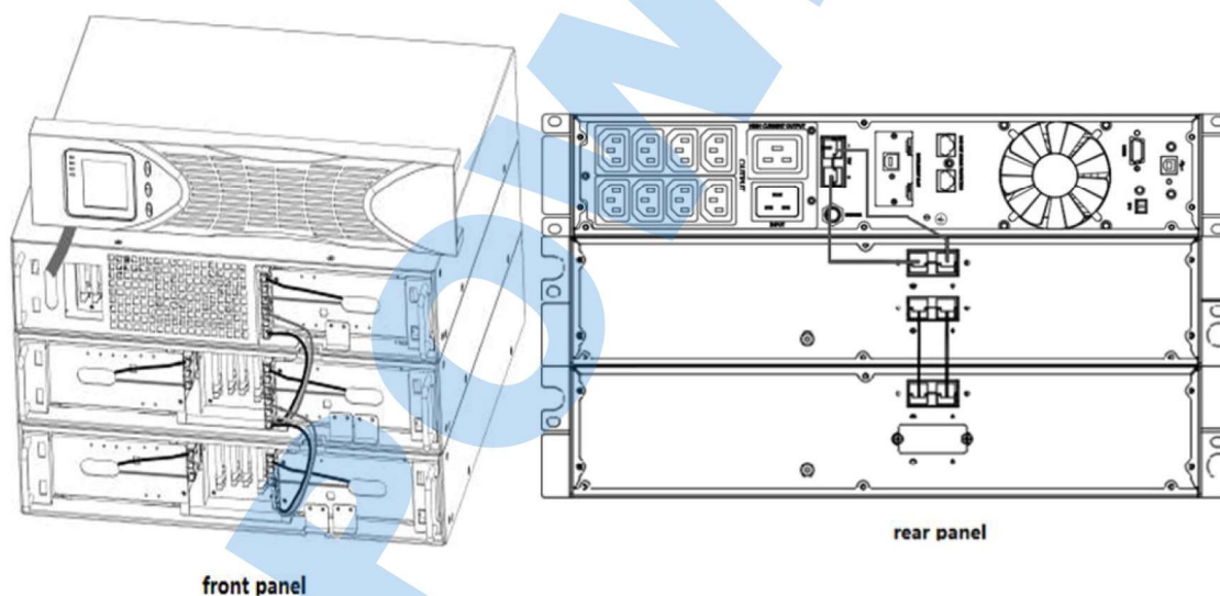
Рис. 5-5. Подключение ББ.
